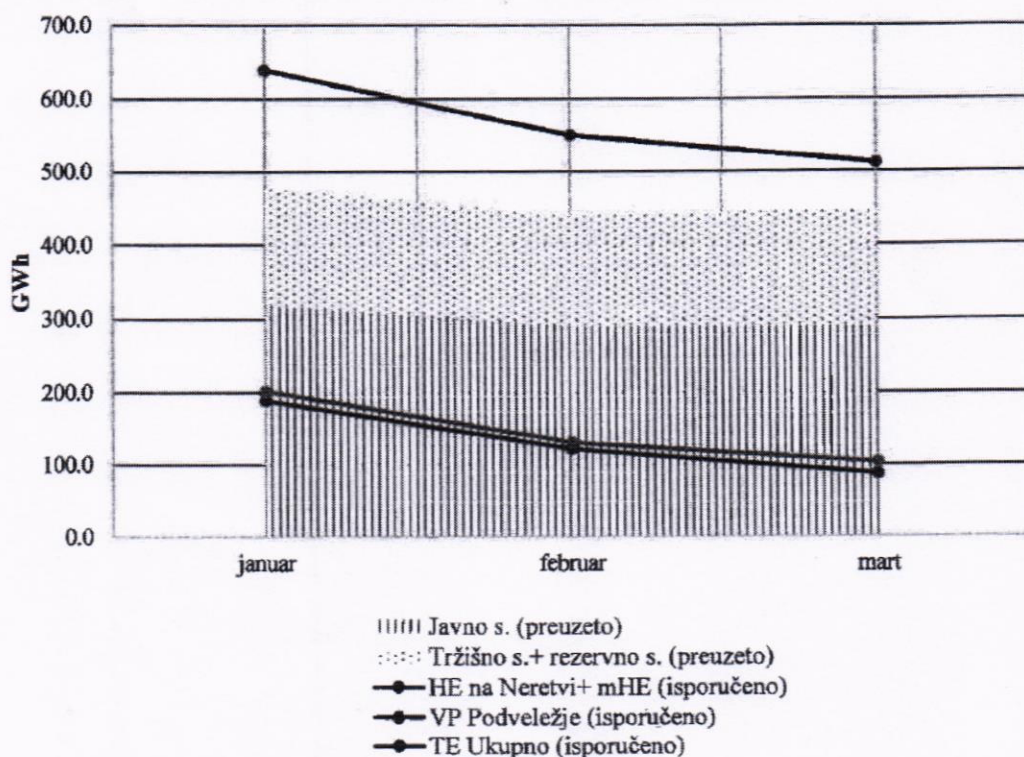
Slika 1 JP Elektroprivreda BiH d.d. - Sarajevo: Ostvarenje proizvodnje i potrošnje električne energije
